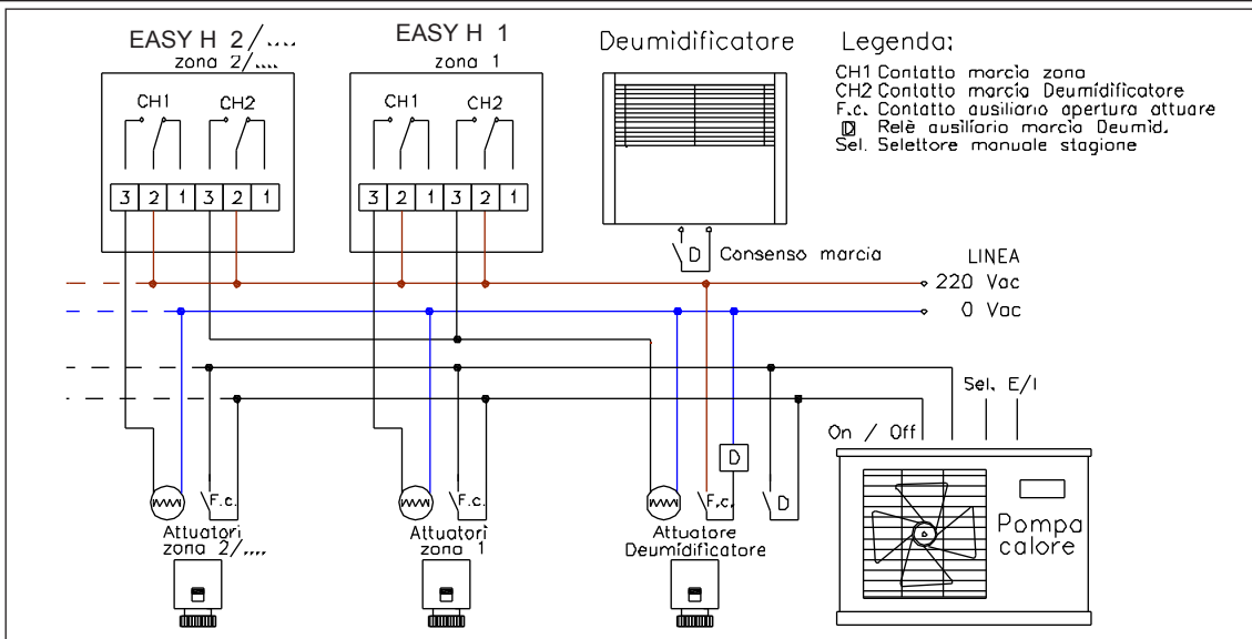
ESEMPIO 1 - Regolazione a più zone termiche in parallelo con 1 deumidificatore e pompa di calore.
