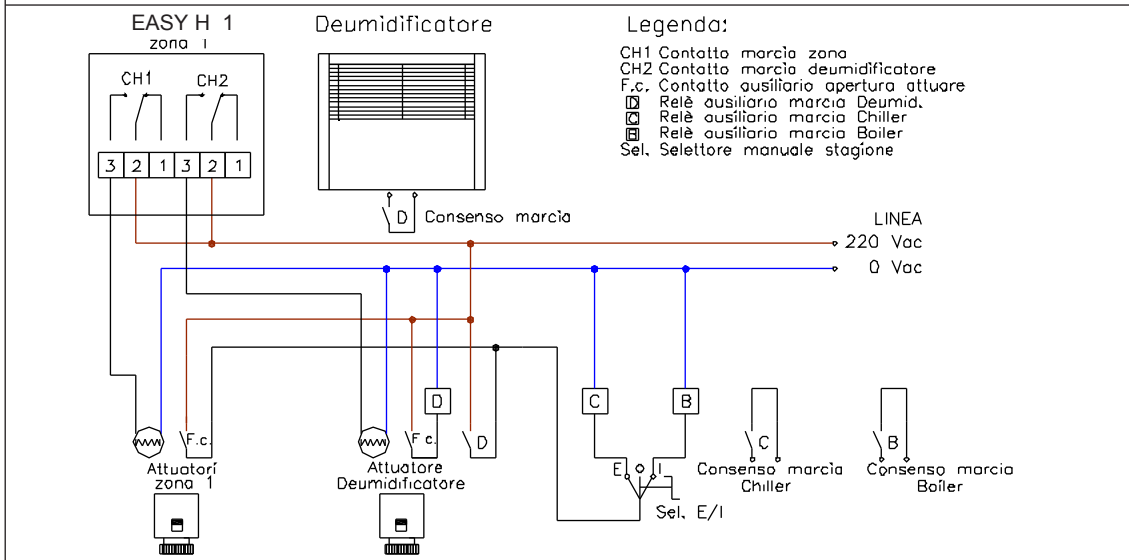
ESEMPIO 2 - Regolazione a una zona termica con 1 deumidificatore e gestione boiler + chiller.
